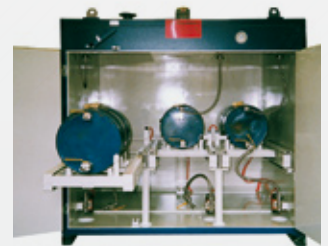
Wärmekammer mit automatischer Abfüllung (Bühne und N 2 -Druck) Heating cabinet with automatical decanting (tilt frame and N 2 pressure)
